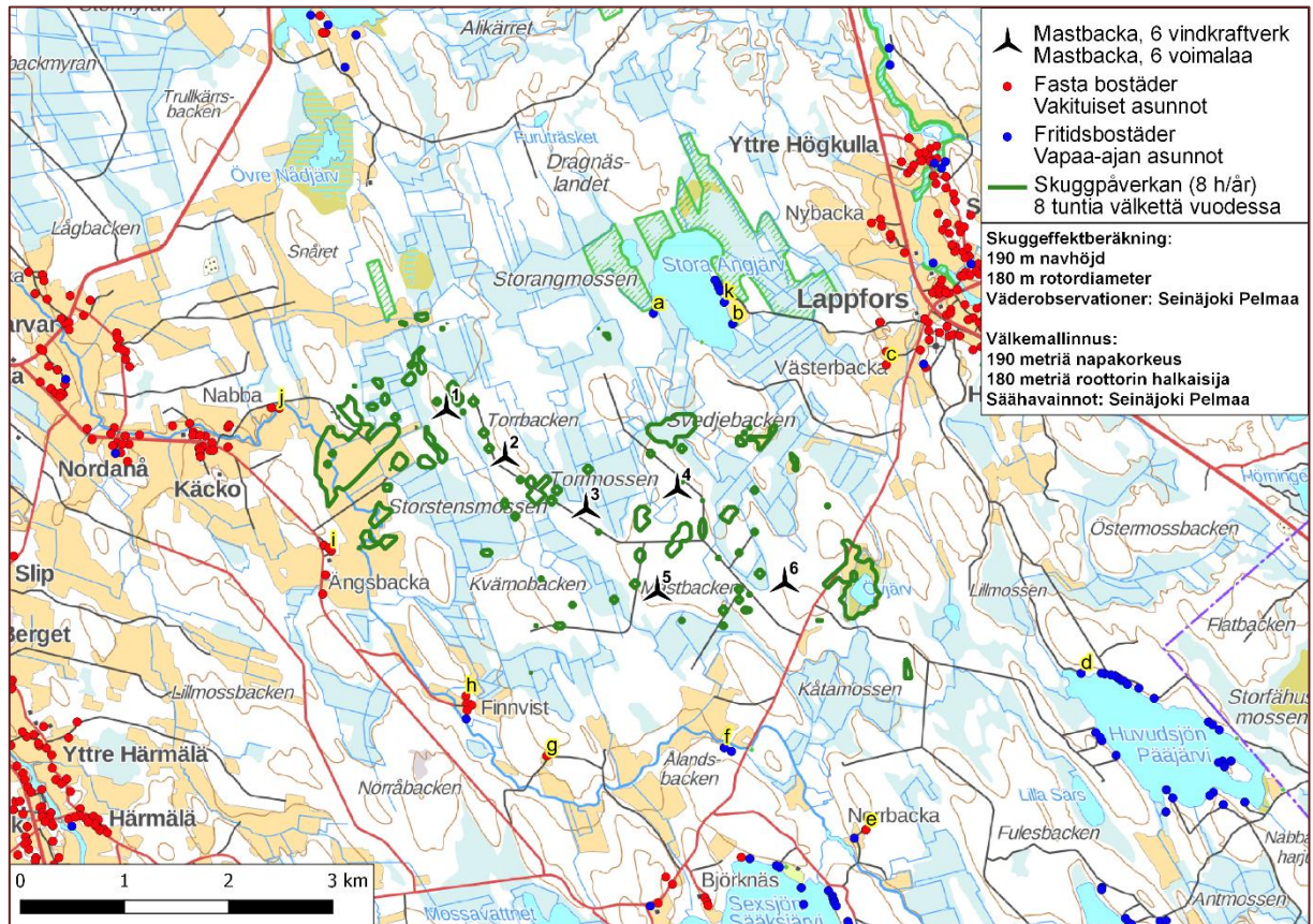
Kuva 3. Skuggeffektpåverkan på Mastbacka vindkraftsområde då skogens inverkan har beaktats. Observationspunkterna har märkts ut i bilden (a-k) och deras skuggnivåer redogörs för i tabell 6.
