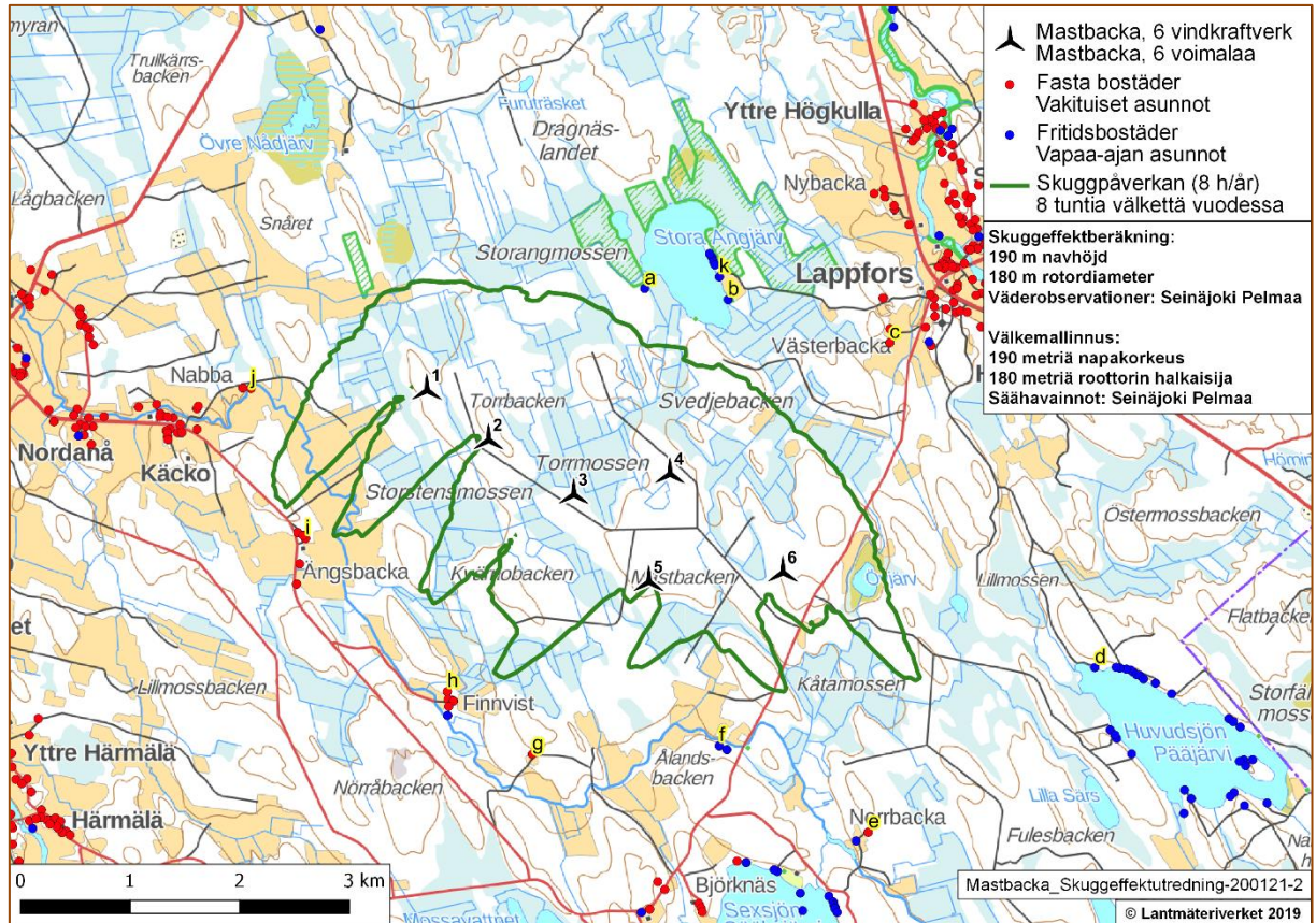
Bild 2. Skuggeffektpåverkan på Mastbacka vindkraftsområde. Observationspunkterna har märkts ut i bilden (a-k) och deras skuggnivåer redogörs för i tabell 5.
